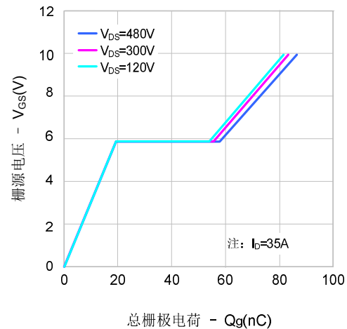
图6. 电荷量特性
