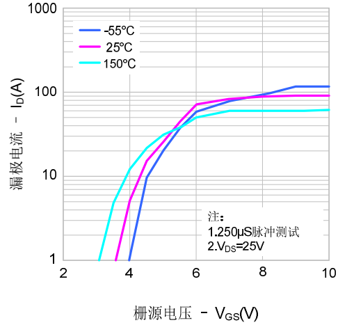
图2. 传输特性
