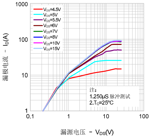
图1. 输出特性
